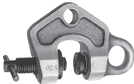
イーグルクランプSBB型規格寸法
